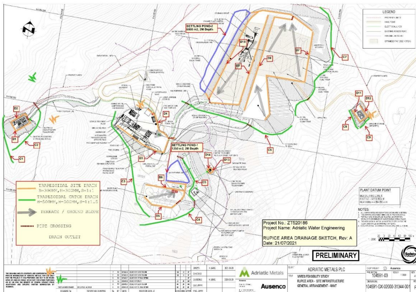
Prikaz 0.16: Elementi odvodnjavanja lokaliteta Rupice
