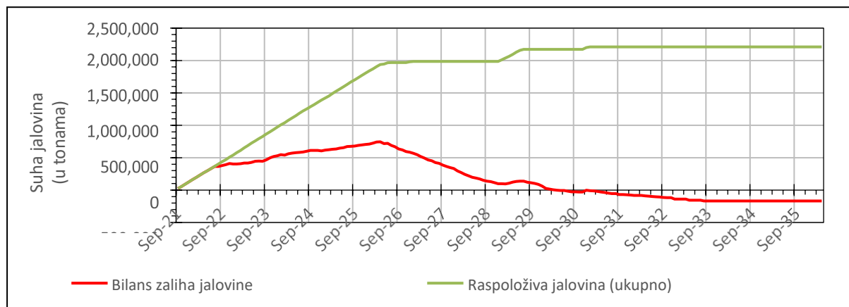
Prikaz 0.11: Bilans zaliha eksploatisanih i transportovanih ruda
