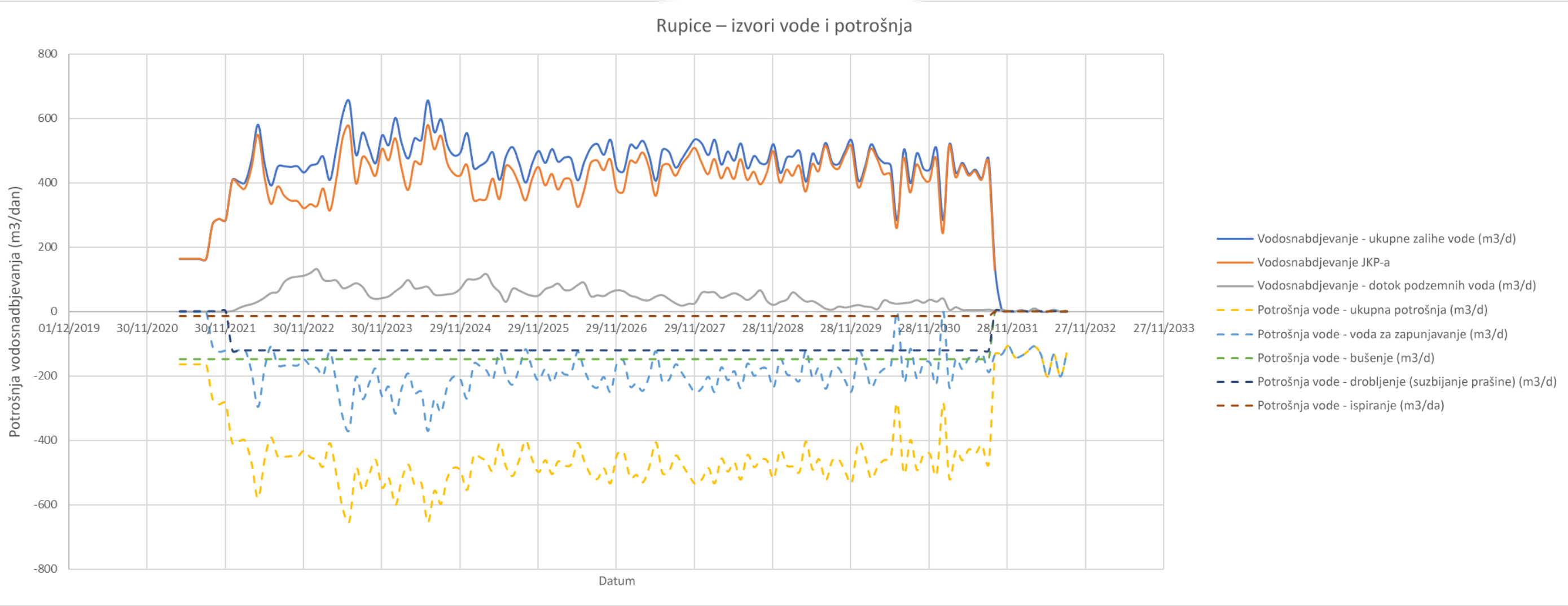
Prikaz 0.15: Bilans snabdijevanja i ispuštanja vode sa lokaliteta Rupice (mjesečno)
